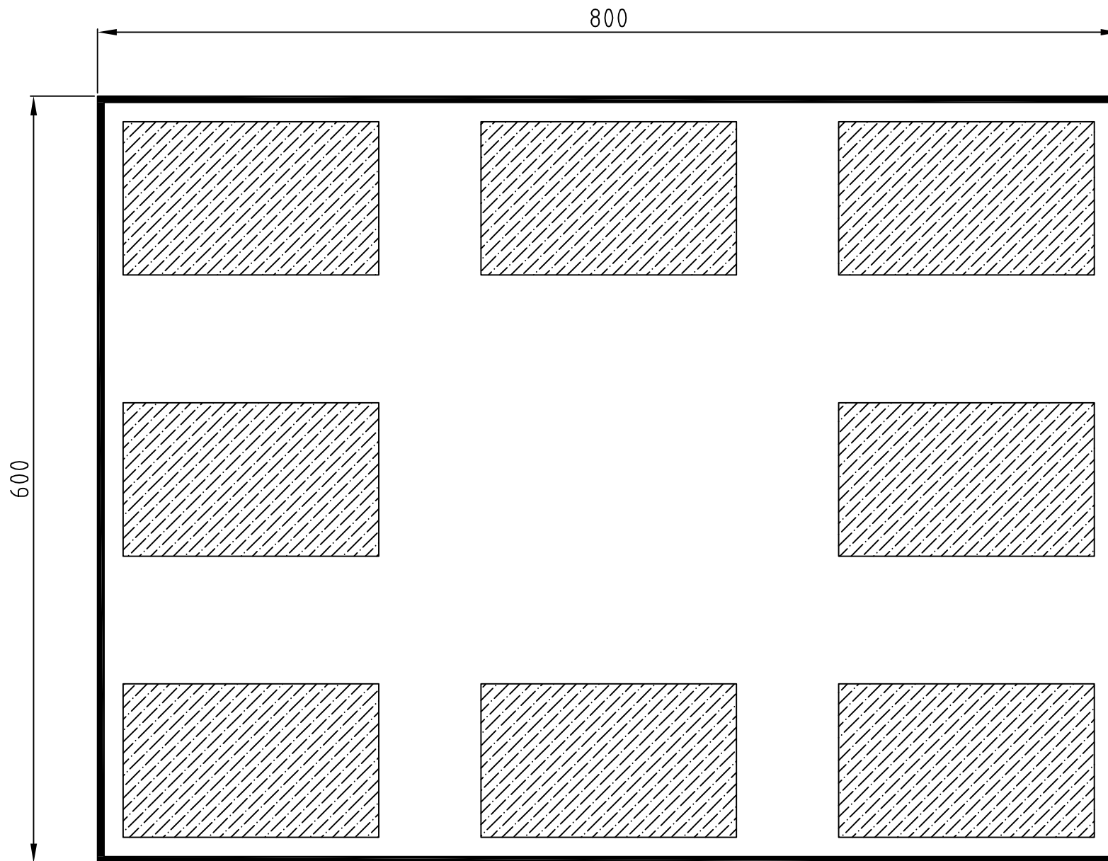
CUUT Ujuvplatform 8x6 m. / 8 x 700L ujukit - kandejõud max 5600 kg.
