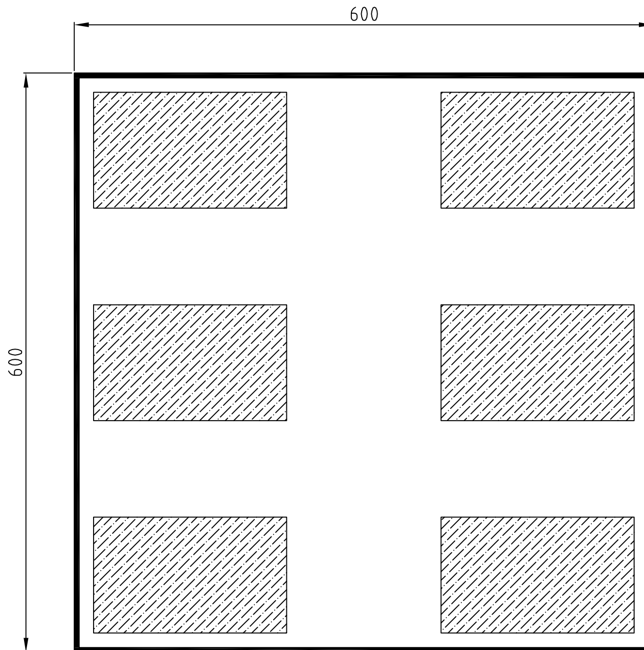
CUUT Ujuvplatform 6x6 m. / 6 x 700L ujukit - kandejõud max 4200 kg.
