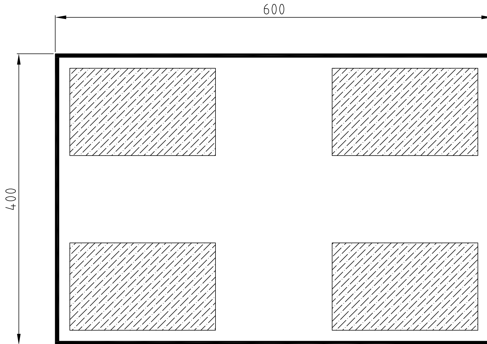
CUUT Ujuvplatform 4x6 m. / 4 x 700L ujukit - kandejõud max 2800 kg.
