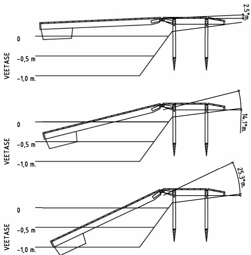
Üheosalise ujusilla kalded veetaseme langusega 0,5m/1,0m
