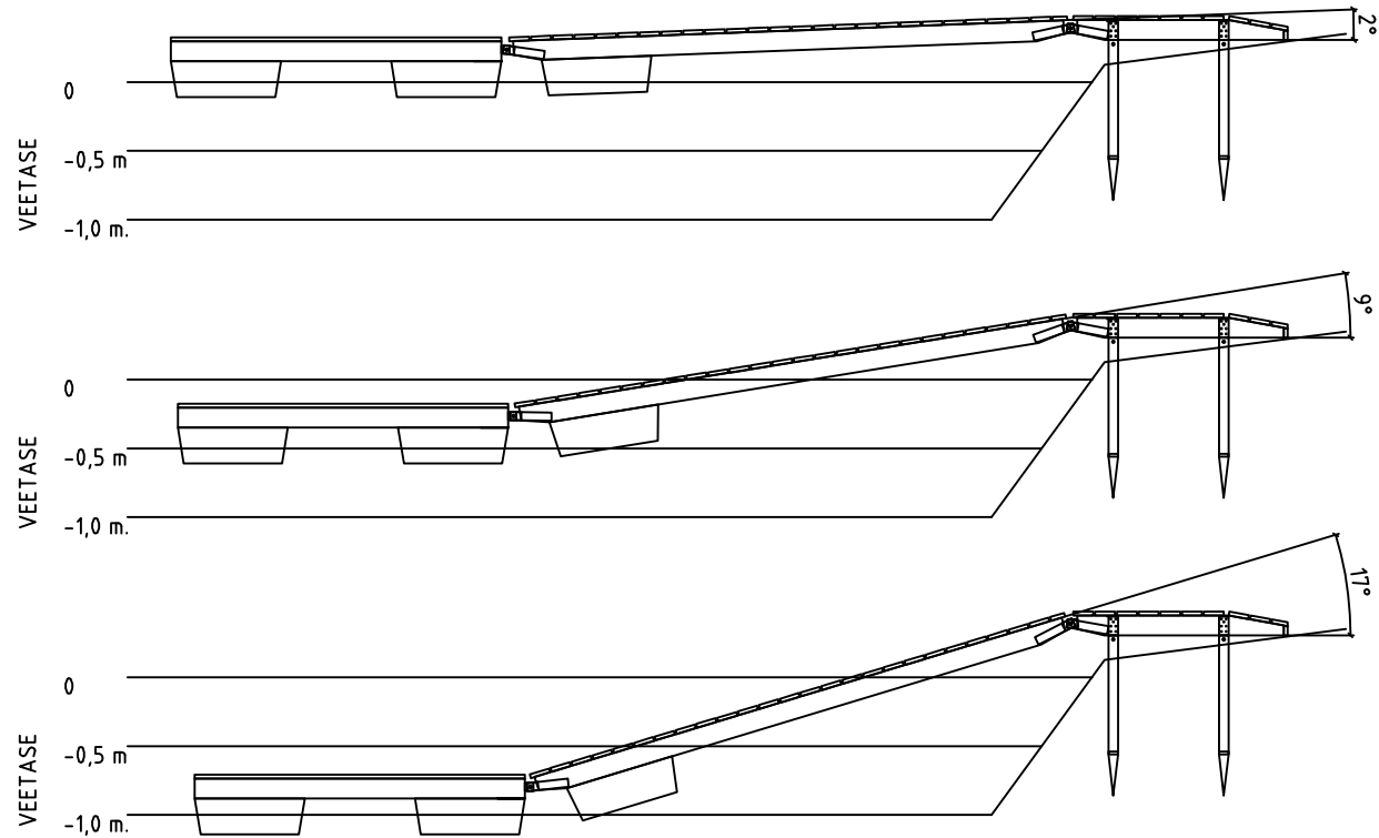
Ujuvplatvormi ja käiguteega sild kalded veetaseme langusega 0,5m/1,0m
