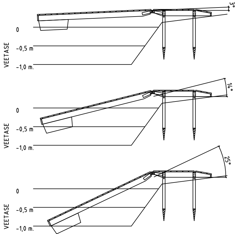
Ühe pontoon ujuki ja käiguteega sild kalded veetaseme langusega 0,5m/1,0m
